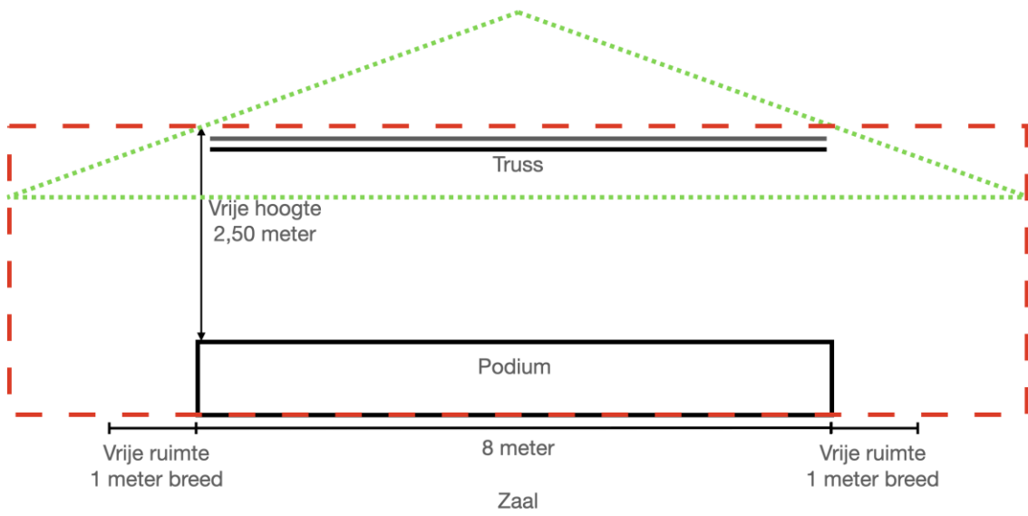
Figuur 2. Vooraanzicht podium PRIME
